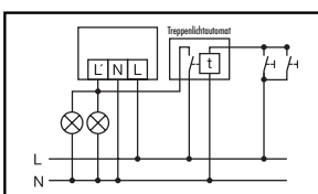
Parallelschaltung und Treppenlichtautomat
