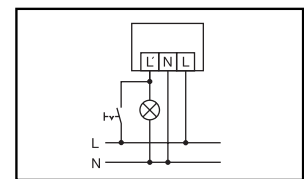
Standardbetrieb mit zusätzlicher Dauerlichtfunktion durch externen Schalter
